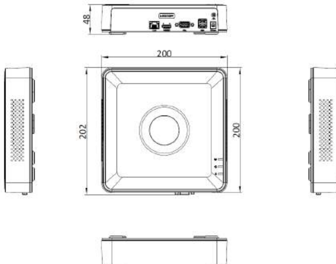
scale/1:1;Unit/mm
