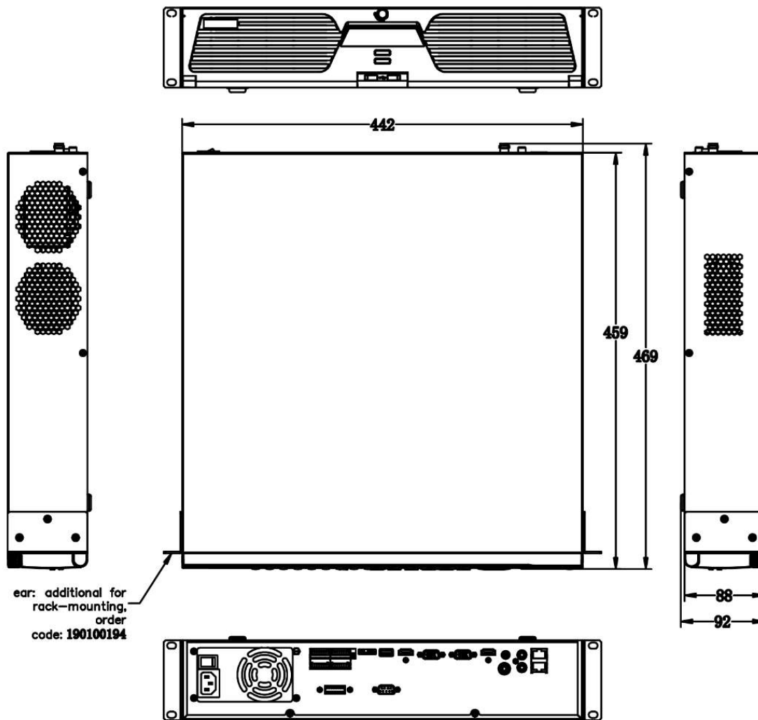
scale/1:1;Unit/mm
